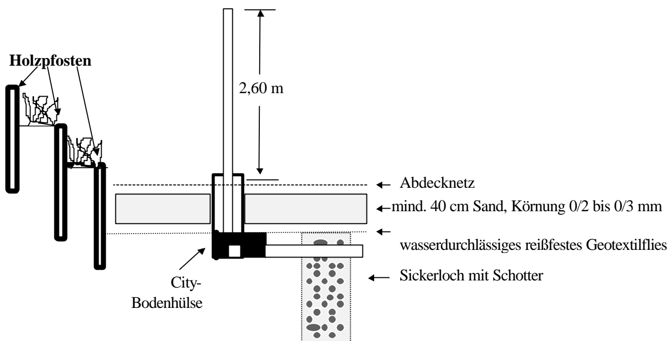
Abb. 2: Querschnitt
